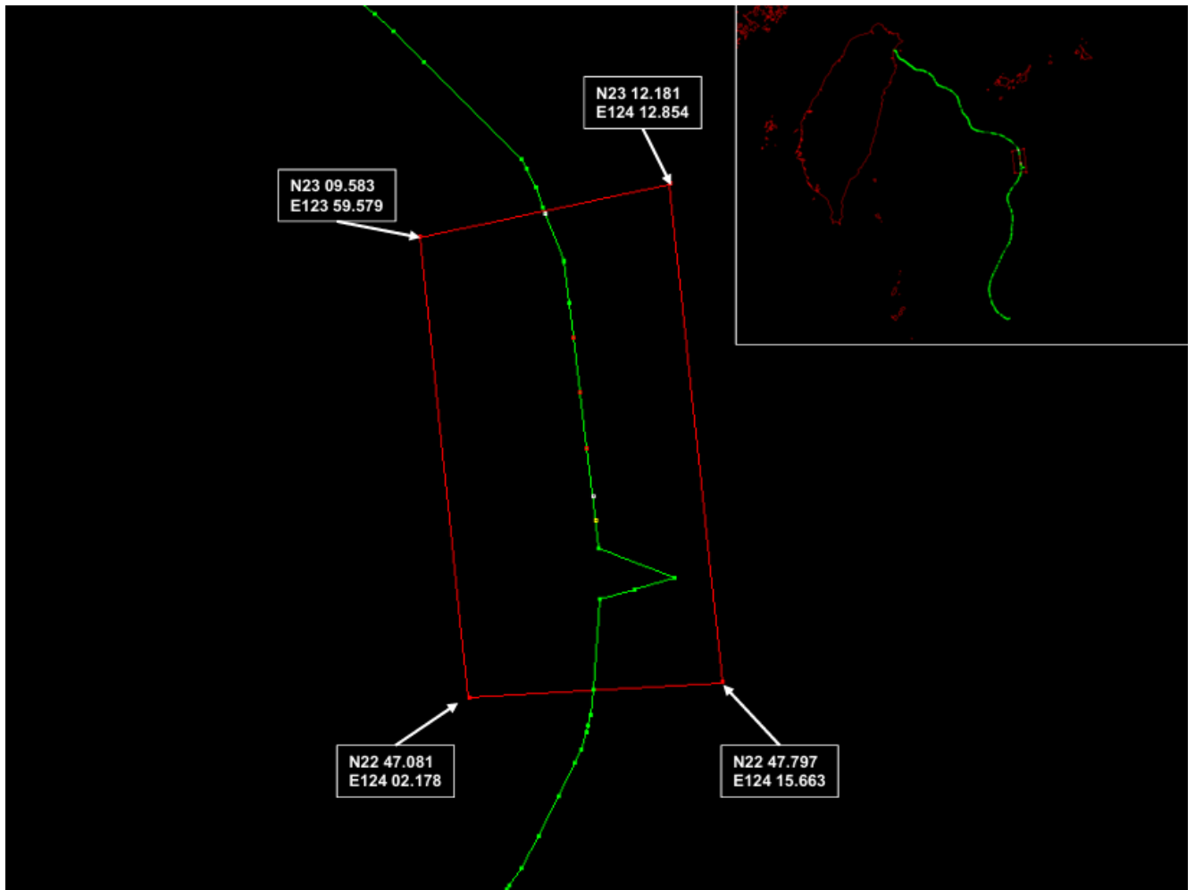
圖二：PLCN S2 海纜故障修理工作範圍
