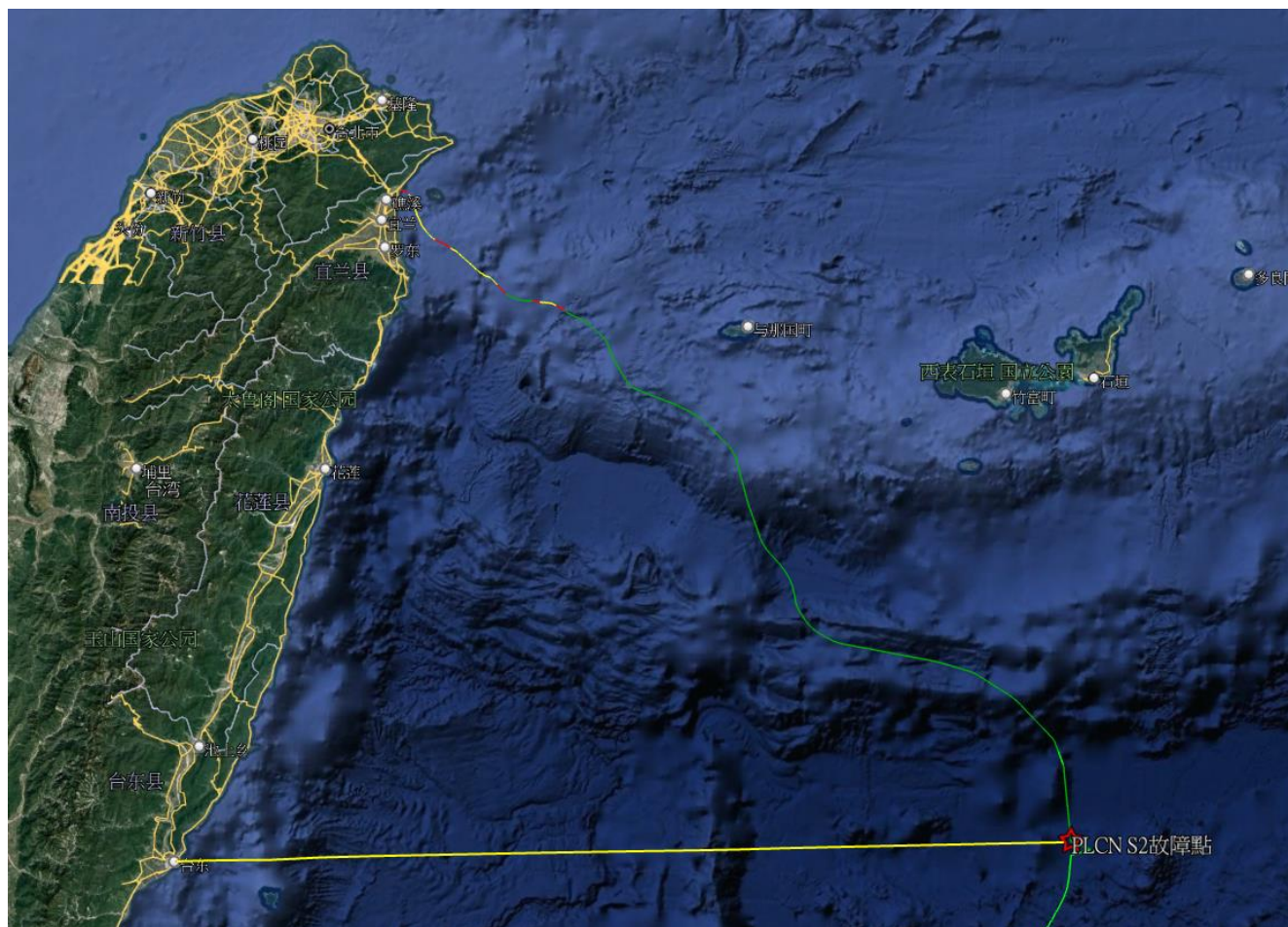
圖一：PLCN S2 區段海纜故障位置圖
