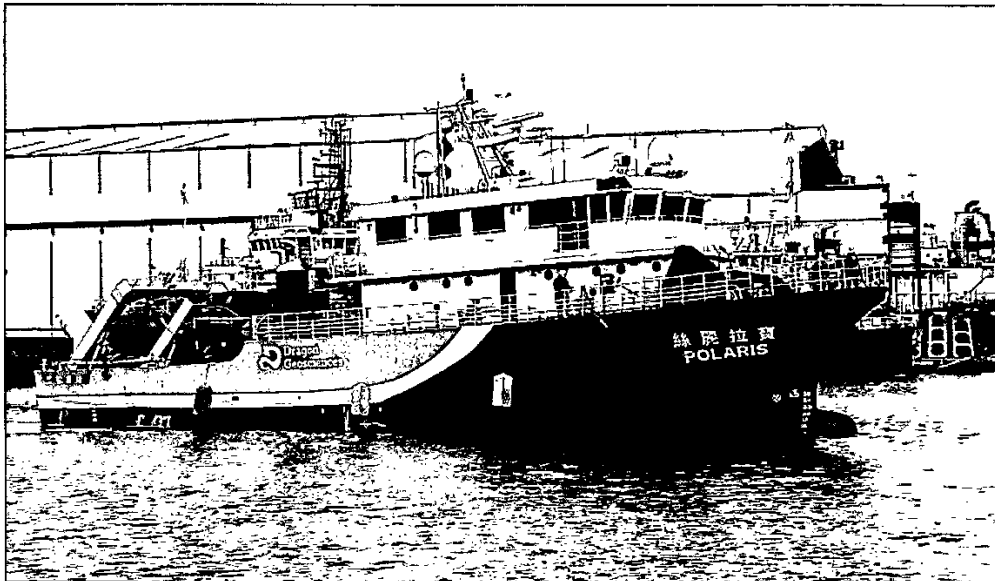
寶拉麗絲右舷照片 (starboard)
