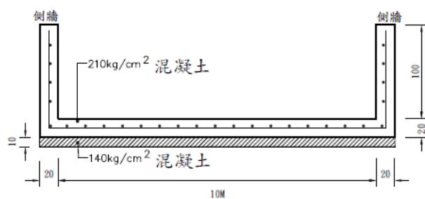
B-B池體渠剖面示意圖
