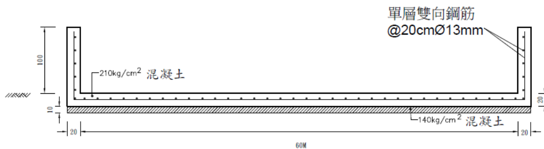
A-A池體剖面示意圖
