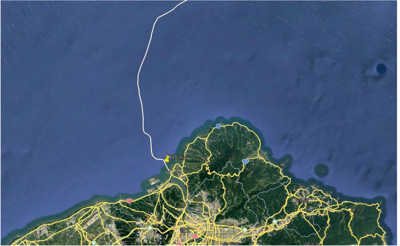
圖一：TPE S4 海纜故障位置圖
