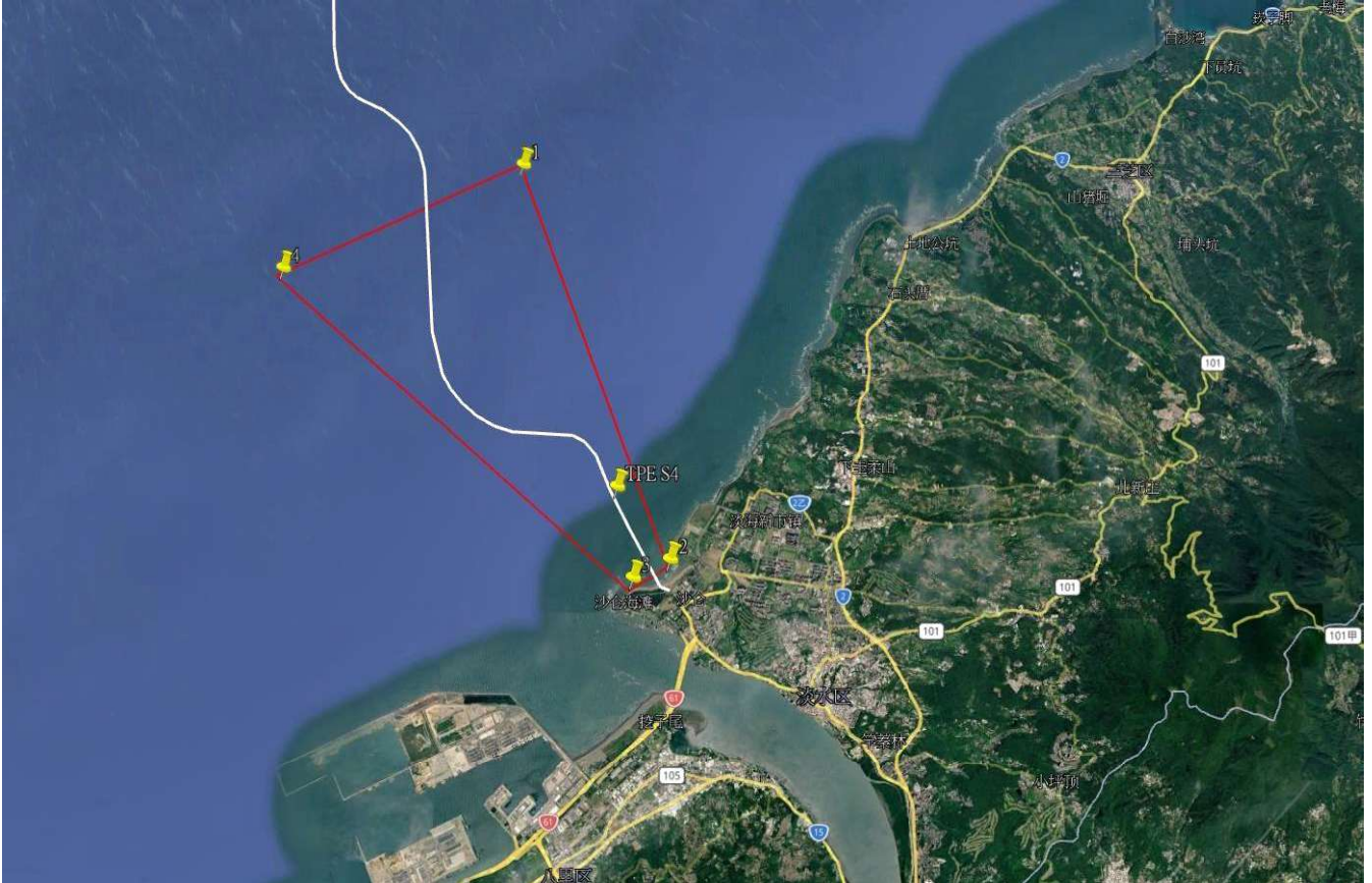
圖二：TPE S4 海纜查勘實際故障位置工作範圍
